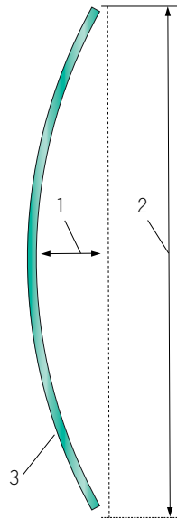
1 Durchbiegung (D) zur Berechnung der generellen Verwerfung t G 2 B oder H, oder die Diagonale 3 Thermisch vorgespanntes Glas
