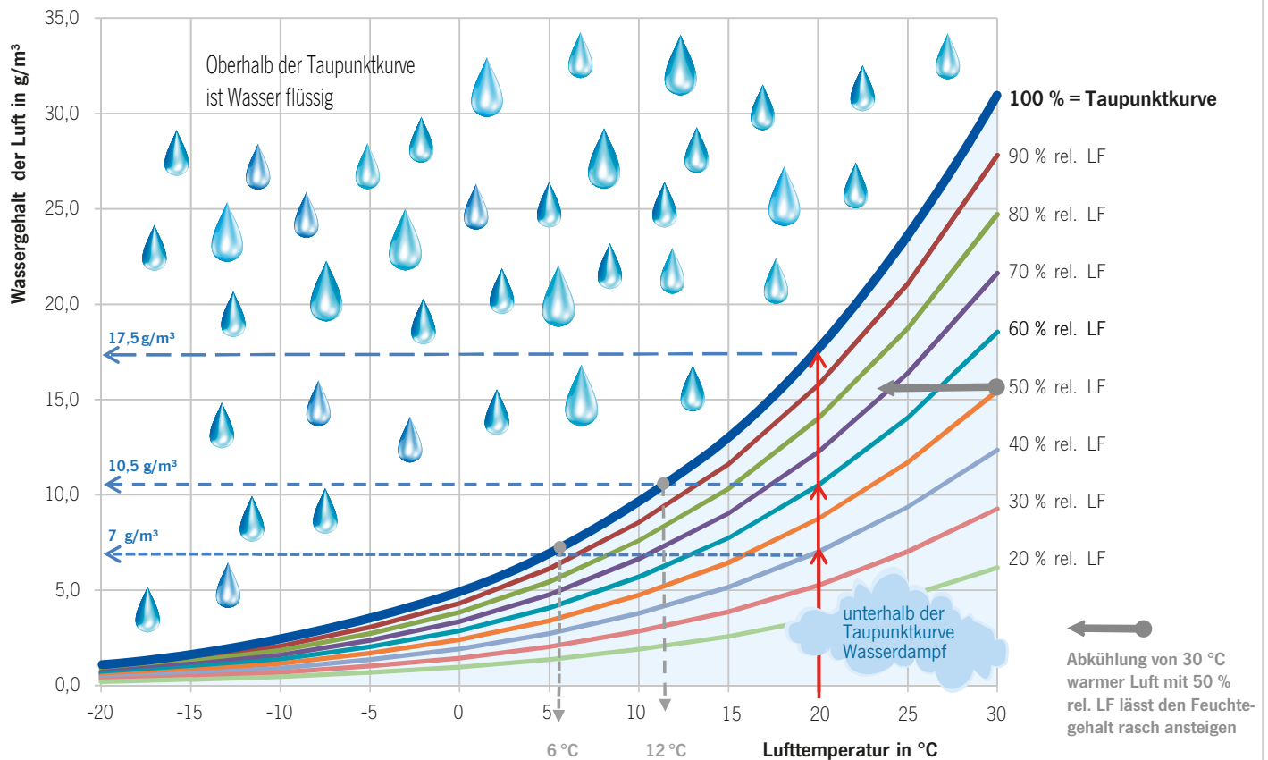
Abbildung: Diagramm mit Kurven gleicher relativer Luftfeuchte in Abhängigkeit von der Temperatur. Die Kurve mit 100 % rel. Luftfeuchte wird Taupunktkurve genannt. Sie gibt den Maximalwert von Feuchtigkeit an, welche die Luft bei einer bestimmten Temperatur bis zur Sättigung aufnehmen kann.
